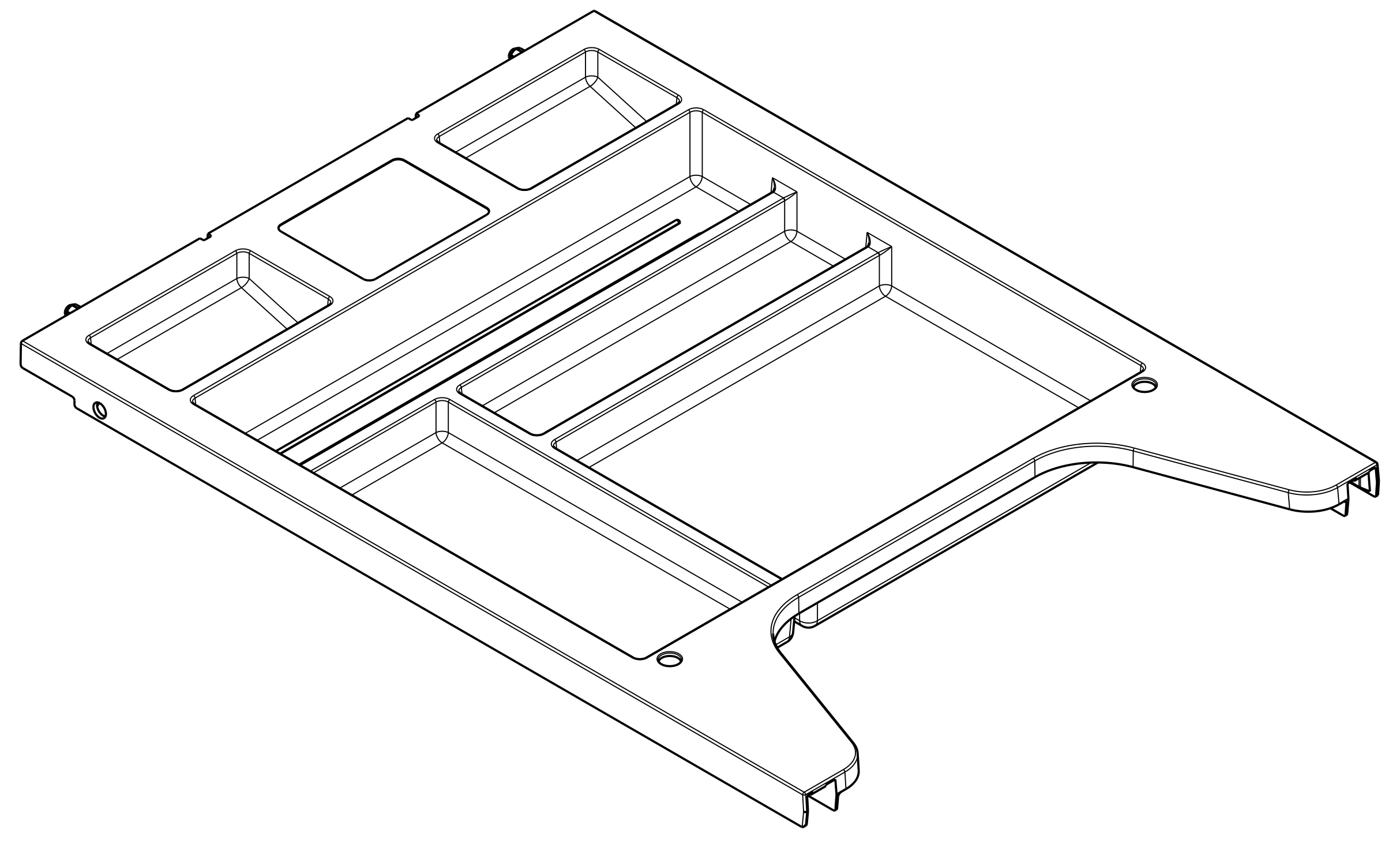
Isometrische Ansicht M 1:2
